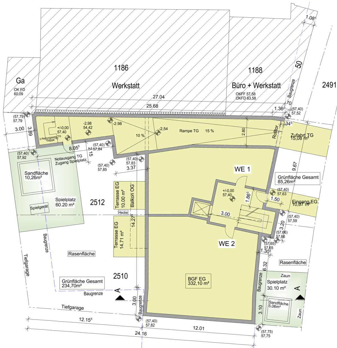
Beispielhafte Aufteilung Grundriss EG
